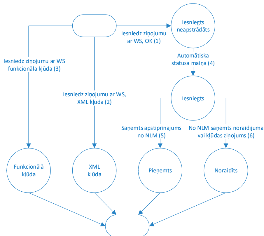
Attēls 158. EMCS KLM VS iesniegto ziņojumu statusi
