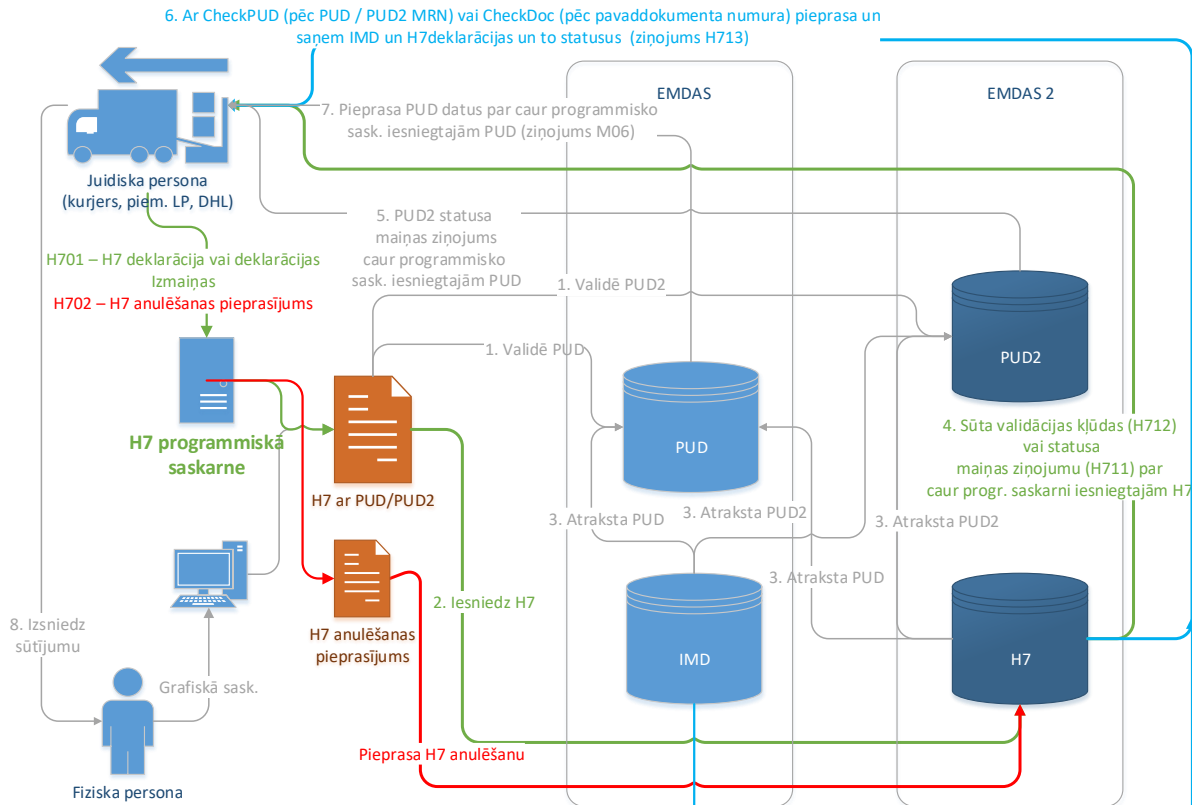
1. attēls. H7 deklarācijas programmiskās saskarnes ziņojumu apmaiņas shēma.
